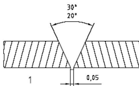
图 1——显示每种类型划线位置的试板
