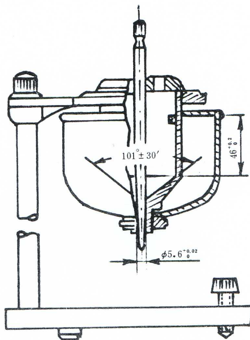
图 1 涂-1 粘度计
