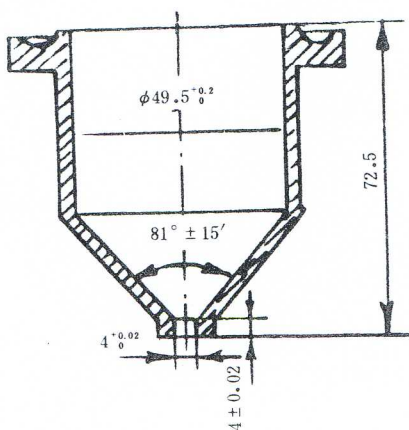
图 2 涂-4 粘度计
