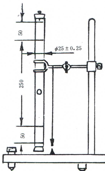
图 3 落球粘度计
