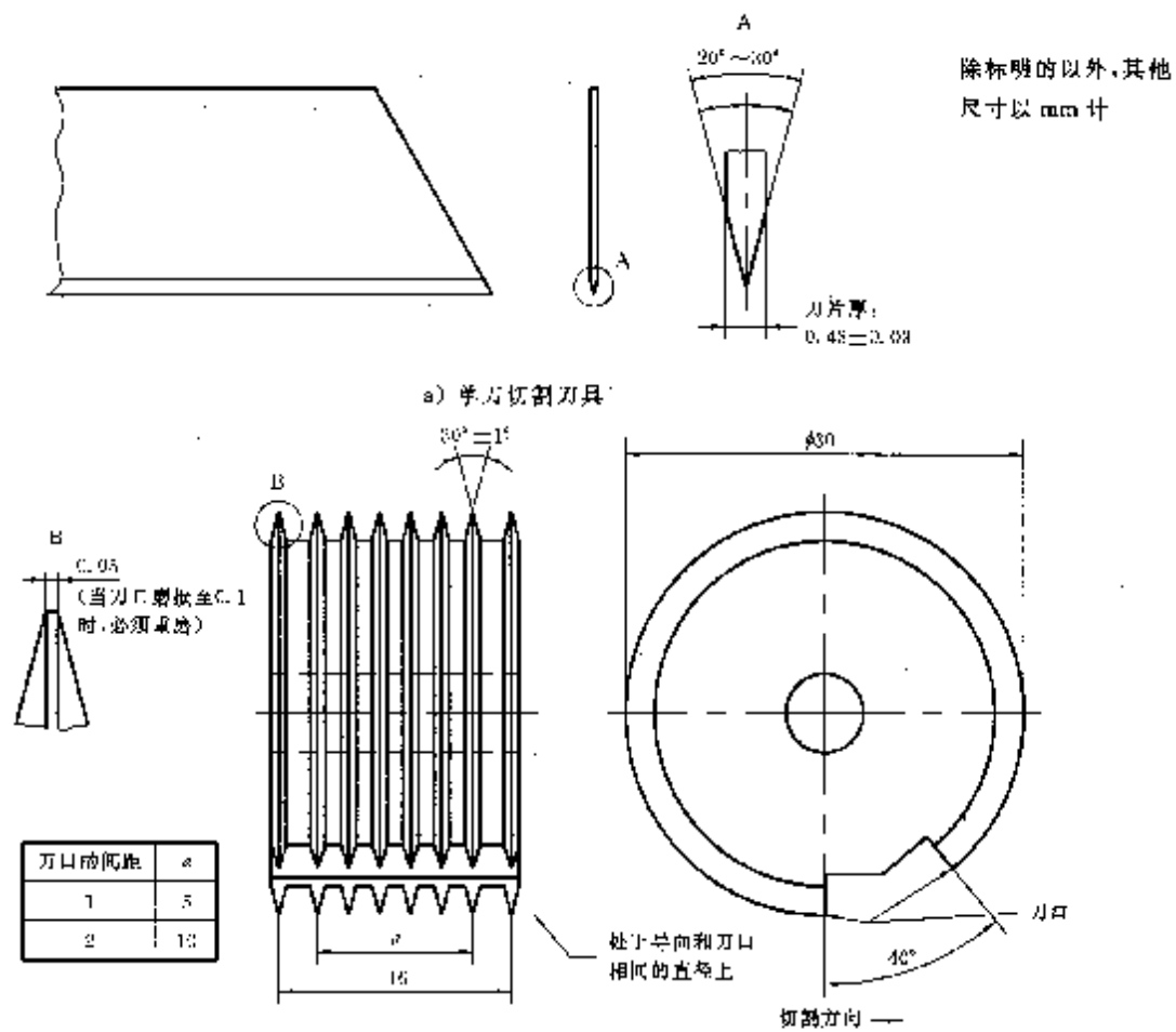
1.2 多刃切削刀具
