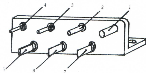
柔韧性测定器
